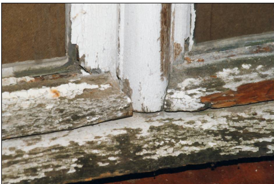
Fig. 4.5. Pièce d'appui et jets d'eau
