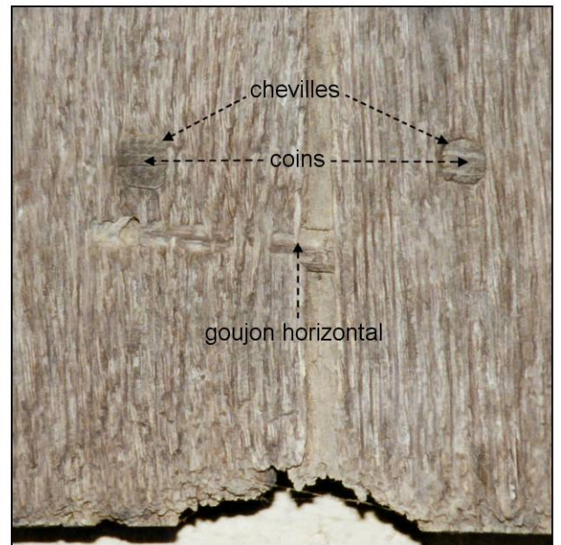
Fig. 3.6. Assemblage du volet (détail)
